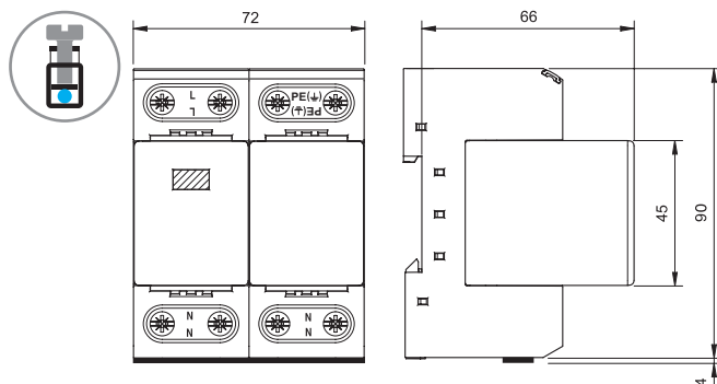
Type 7P.02 Bornes à cage
