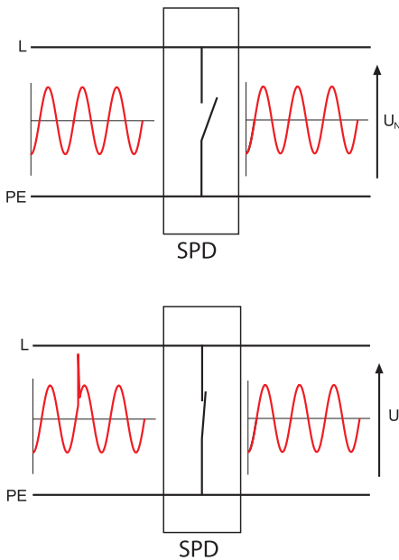
Figure 1 : fonctionnement idéal d'un parafoudre
