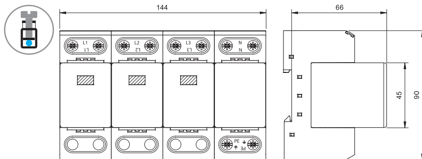
Type 7P.04 Bornes à cage
