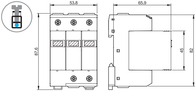
Types 7P.23.8 / 7P.43 Bornes à cage
