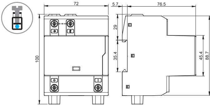
Type 7P.13.9.000.x006 Bornes à cage
