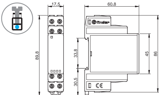
Type 7P.37.8.275.1003 Bornes à cage
