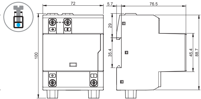
Type 7P.13.9.500.x006 Bornes à cage
