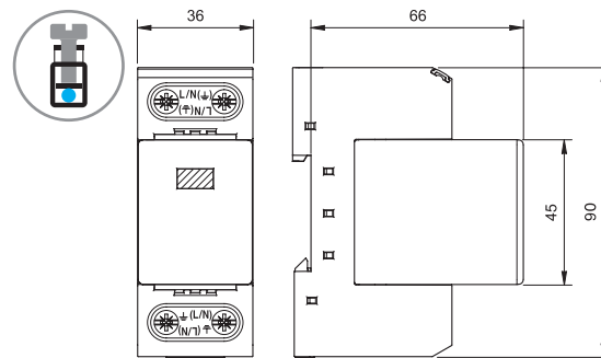
Type 7P.01 Bornes à cage
