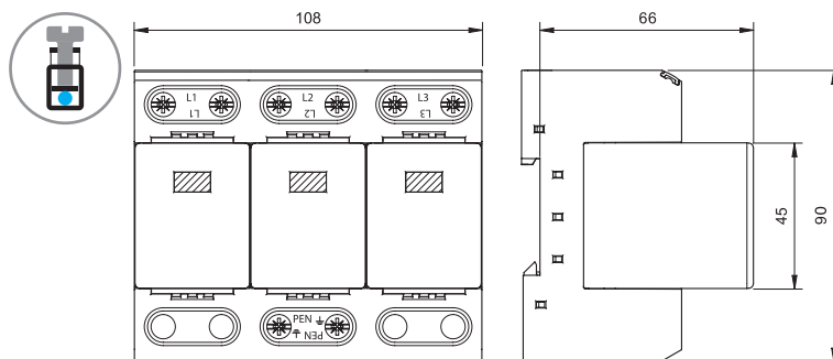
Type 7P.03 Bornes à cage
