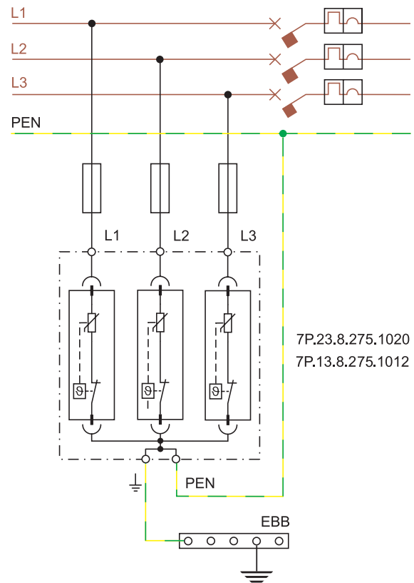
TN-C TRIPHASÉ EN AMONT DE LA PROTECTION
