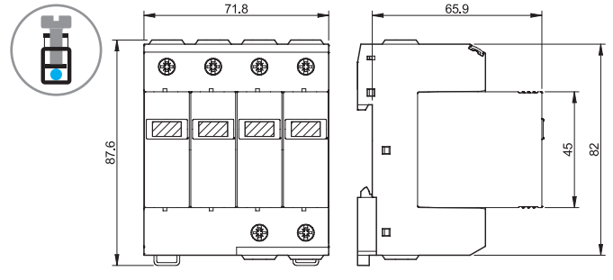
Types 7P.25 / 7P.45 Bornes à cage
