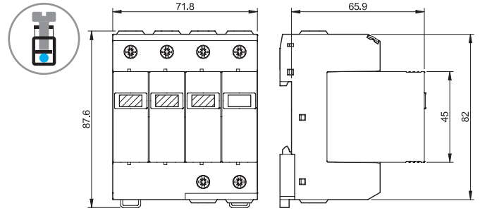
Types 7P.24 / 7P.44 Bornes à cage
