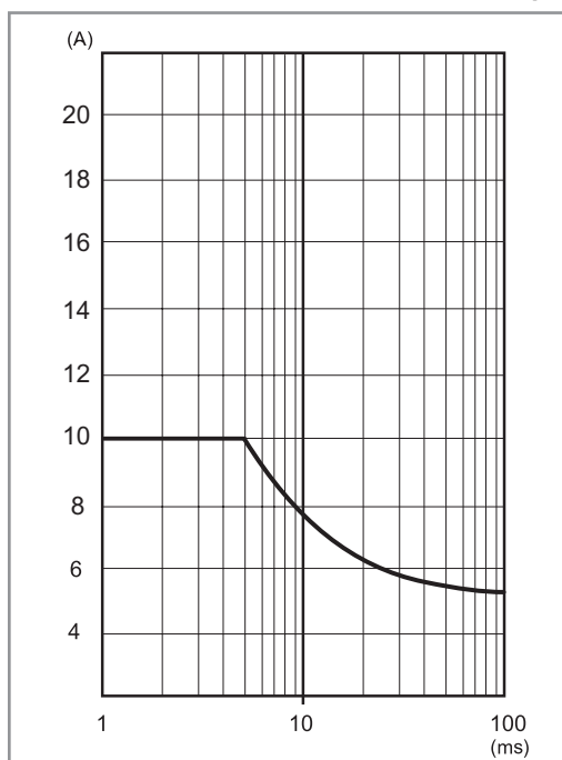
P78-8 Pic de courant en sortie en fonction du temps (78.1D)
