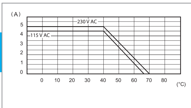
L78-7 Courant de sortie en fonction de la température ambiante (78.1B)
