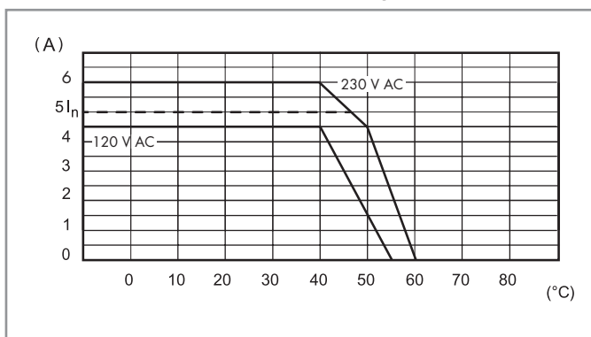
L78-6 Courant de sortie en fonction de la température ambiante (78.1A)
