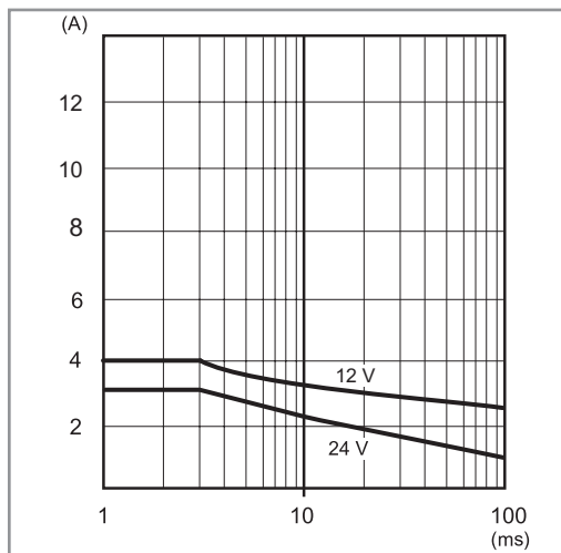
P78-3 Pic de courant en sortie en fonction du temps (78.36) 12 V
