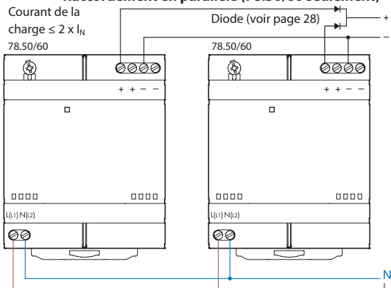
Raccordement en parallèle (78.50/60 seulement)
