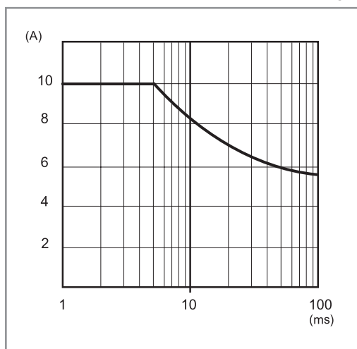
P78-6 Pic de courant en sortie en fonction du temps (78.1A)
