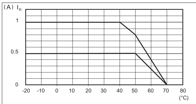
L78-1 Courant de sortie en fonction de la température ambiante (78.12) 24 V
