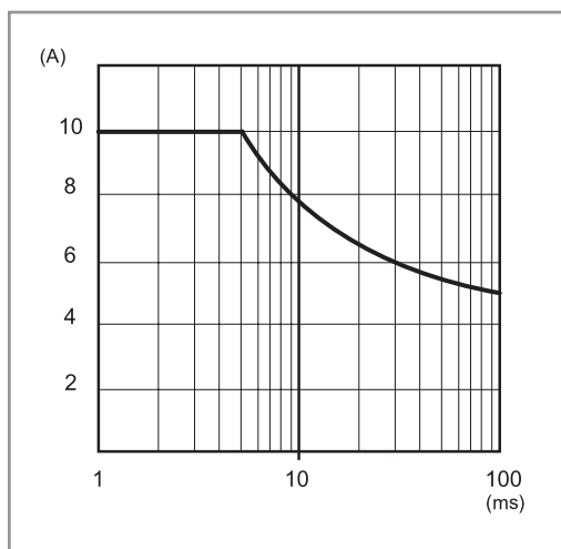
P78-8 Pic de courant en sortie en fonction du temps (78.1D)
