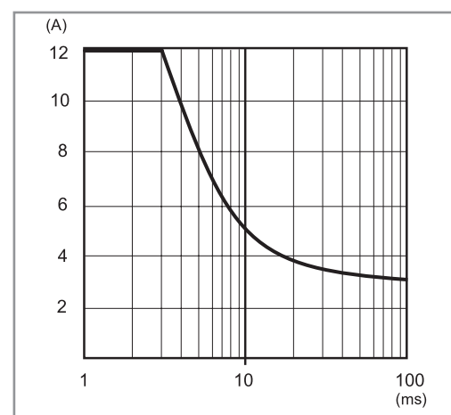
P78-3 Pic de courant en sortie en fonction du temps (78.36) 12 V
