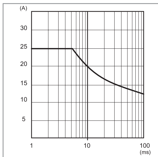
P78-10 Pic de courant en sortie en fonction du temps (78.2E)
