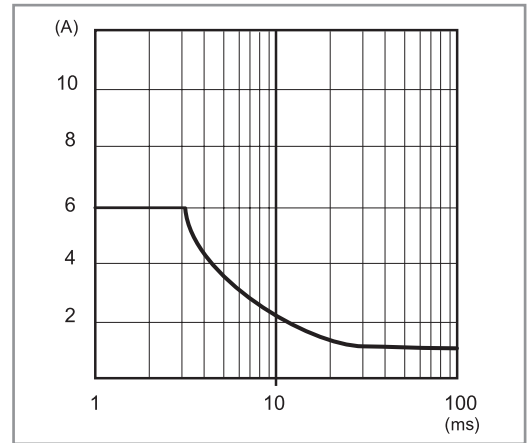
P78-4 Pic de courant en sortie en fonction du temps (78.60)
