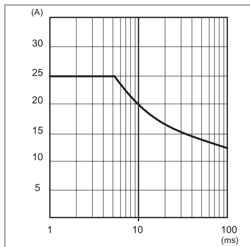
P78-9 Pic de courant en sortie en fonction du temps(78.2A)
