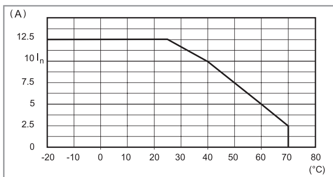
L78-10 Courant de sortie en fonction de la température ambiante (78.2E)
