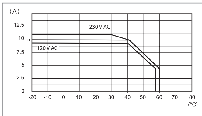
L78-9 Courant de sortie en fonction de la température ambiante (78.2A)
