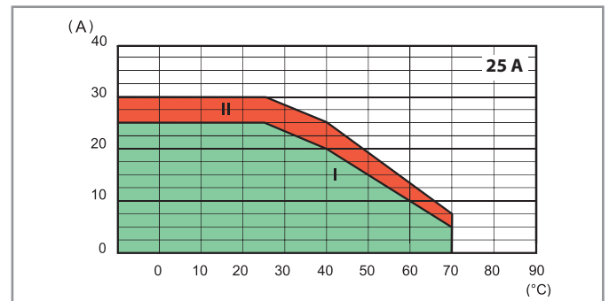
L77-6 Courant RMS en fonction de la température ambiante - 77.21.x.xxx.825x
