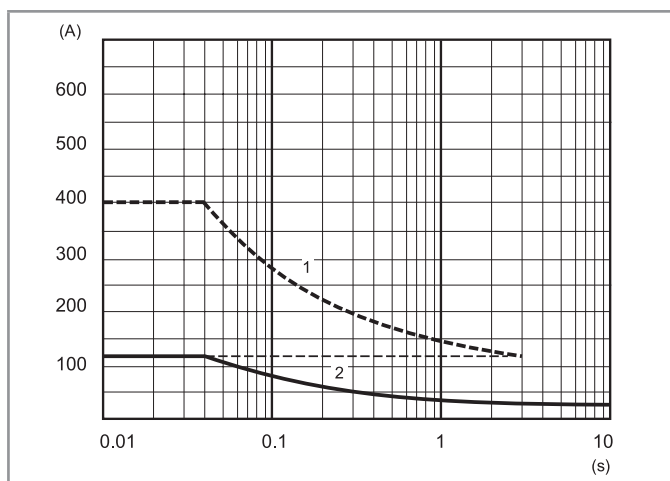
L77-10 Pic de courant (AC) en fonction du temps
