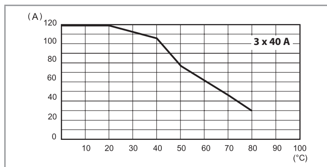
L77-23 Courant RMS en fonction de la température ambiante 77.B3.x.xxx.8671
