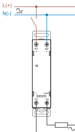
Connexion monophasée (77.31...805x)
