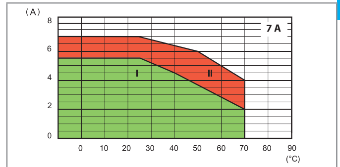
L77-4 Courant efficace maximum DC en fonction de la température ambiante - 77.01.9.024.9125 - Circuit d'entrée 32 V DC
