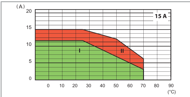
L77-3 Courant efficace maximum DC en fonction de la température ambiante - 77.01.9.024.9024 - Circuit d'entrée 32 V DC
