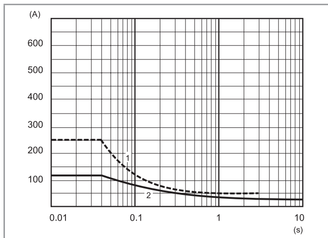
L77-11 Pic de courant (AC) en fonction du temps
