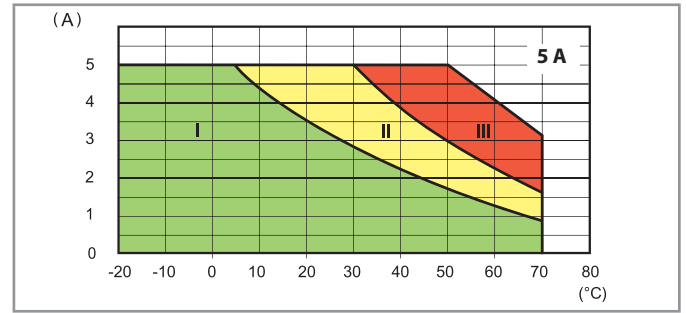
L77-2 Courant efficace maximum AC en fonction de la température ambiante - 77.01.8.230.805x - Circuit d'entrée 265 V AC
