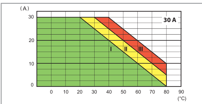
L77-7 Courant RMS en fonction de la température ambiante - 77.31.x.xxx.80xx
