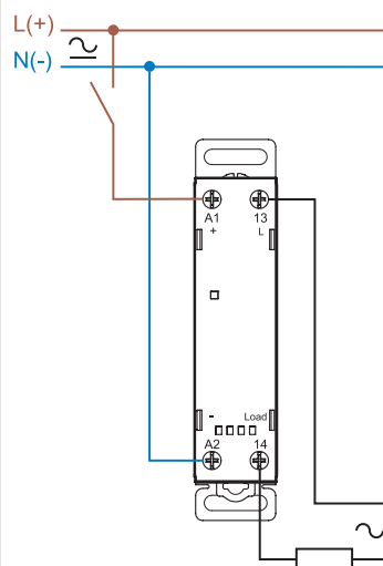
Connexion monophasée (77.31...807x)
