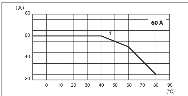
L77-15 Courant RMS en fonction de la température ambiante 77.D1.x.xxx.8x50
