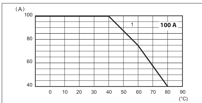
L77-17 Courant RMS en fonction de la température ambiante 77.G1.x.xxx.8x50
