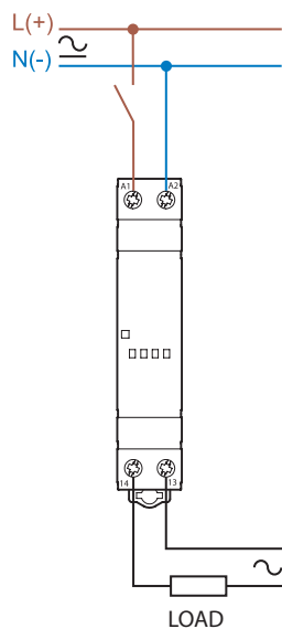
Connexion monophasée (77.01...805x)
