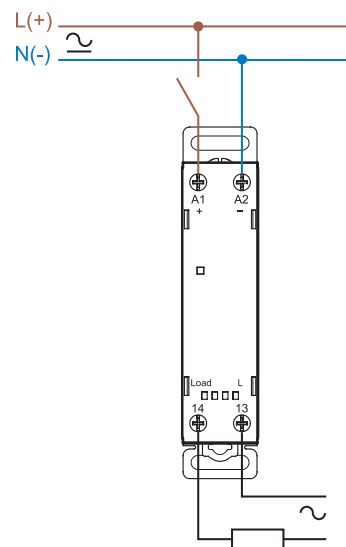
Connexion monophasée (77.11/77.21)
