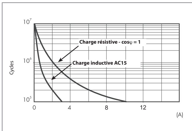
F 40.6 - Durée de vie électrique (AC) en fonction de la charge Type 40.62
