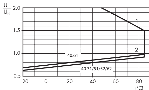
R 40 - Plage de fonctionnement bobine DC en fonction de la température ambiante - Bobine sensible, types 40.31/51/52/61/62
