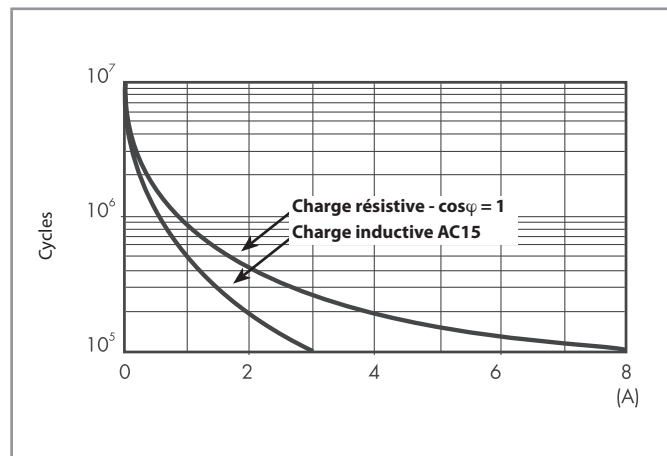
F 40.2 - Durée de vie électrique (AC) en fonction de la charge Type 40.52
