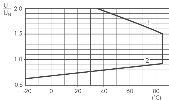
R 40 - Plage de fonctionnement bobine AC en fonction de la température ambiante
