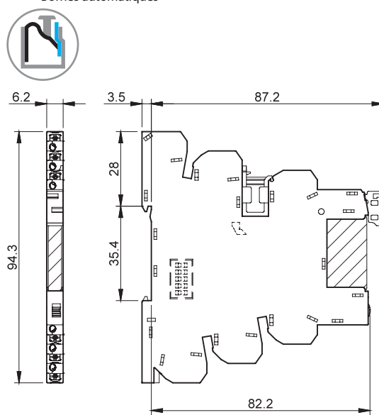
Types 39.90 39.91 Bornes automatiques
