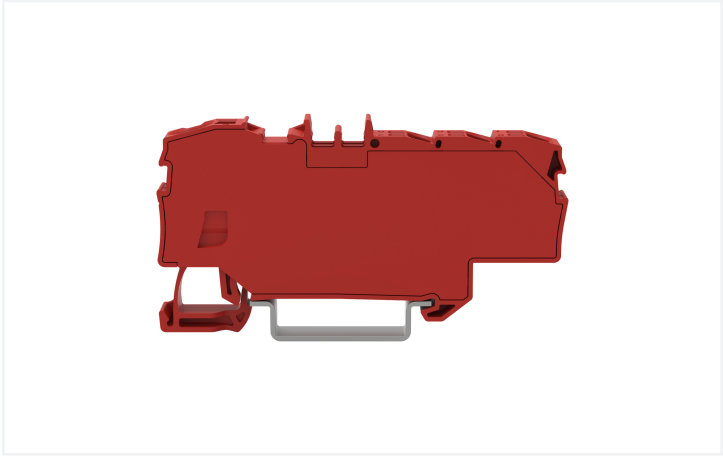
Borne de distribution série 2006 avec Push-in CAGE CLAMP®
