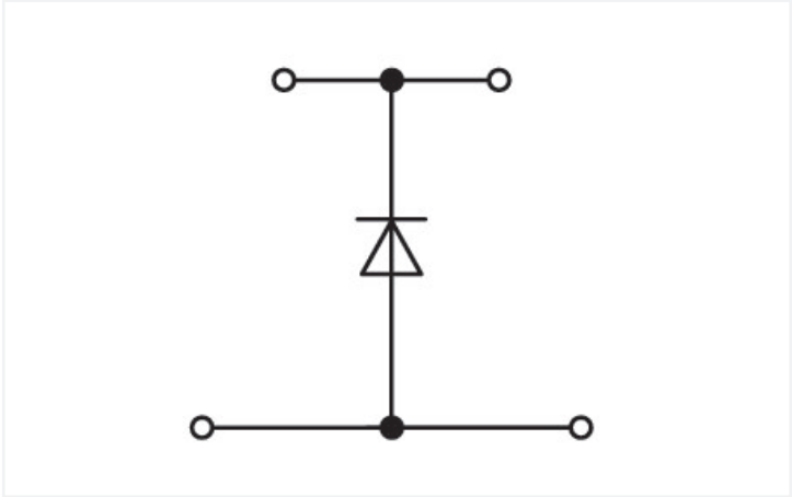
Borne à deux étages série 2002, gris
