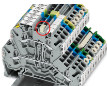
Contact de pontage vertical à deux étages (2002-492), connecté, pour pontage sur deux étages.
