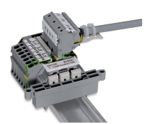
Bloc de bornes, connexion d'un moteur
