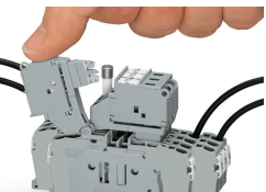
Borne à fusible avec porte fusible pivotant Faire pivoter le porte-fusible jusqu'au cran d'arrêt
