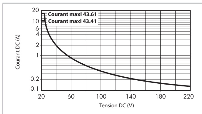
H 43 - Pouvoir de coupure maxi pour une charge en DC1
