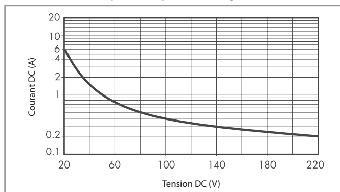
H 32 - Pouvoir de coupure maxi pour une charge en DC1
